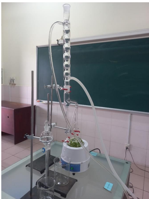
Hình ảnh về thí nghiệm chưng cất tinh dầu bằng phương pháp lôi cuốn hơi nước.
